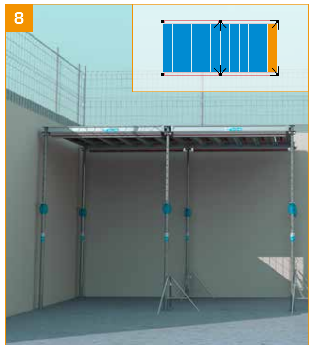
- Die Schritte 5 bis 7 wiederholen und die Installation der Paneele Eco+ so nahe wie möglich an der Wand beenden.
