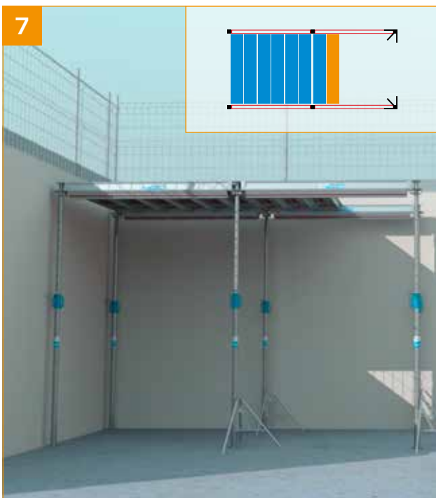
- Mit der Installation der Eco+ Paneele fortfahren wie in den Schritten 2 bis 4 angegeben.
