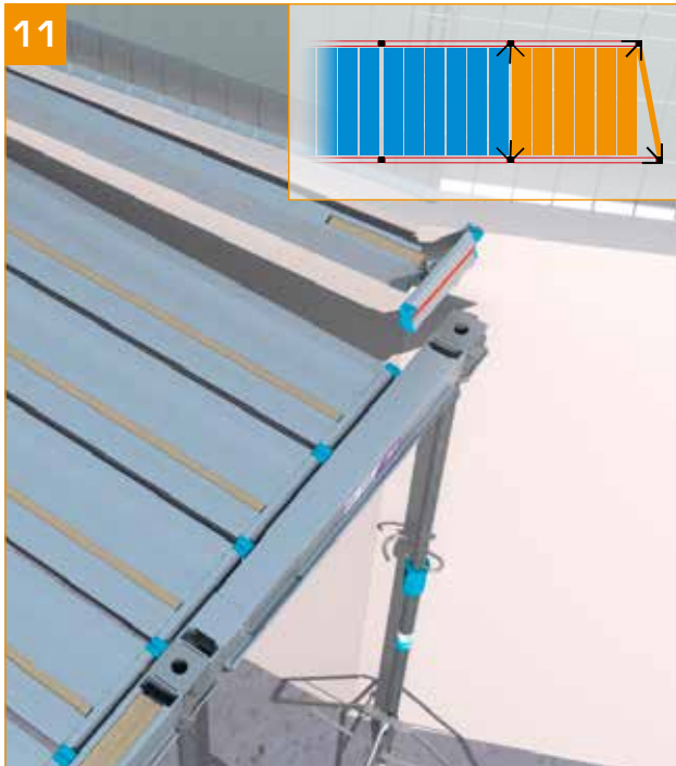
- Den ausziehbaren Nebenträger für Verlegung im Winkel anbringen.
