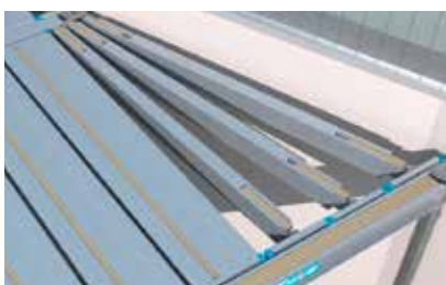
Die ausziehbaren Träger ermöglichen eine bessere Anpassung an die Randbereiche des Abschnitts
