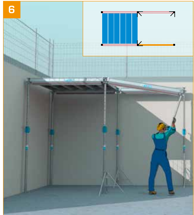
- Der Monteur verwendet die Stütze, um den Hauptträger zu platzieren. - Die Stabilität provisorisch mit Dreibeinen sicherstellen.
